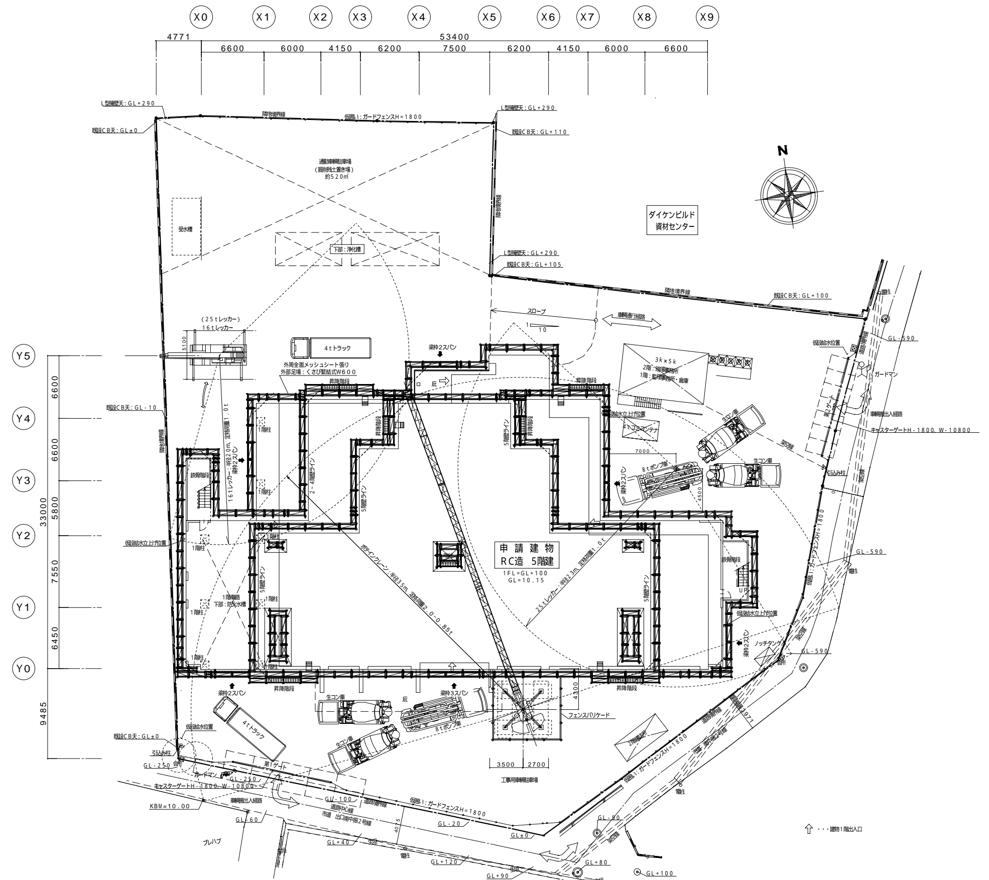
総合仮設計画図 S=1/200
