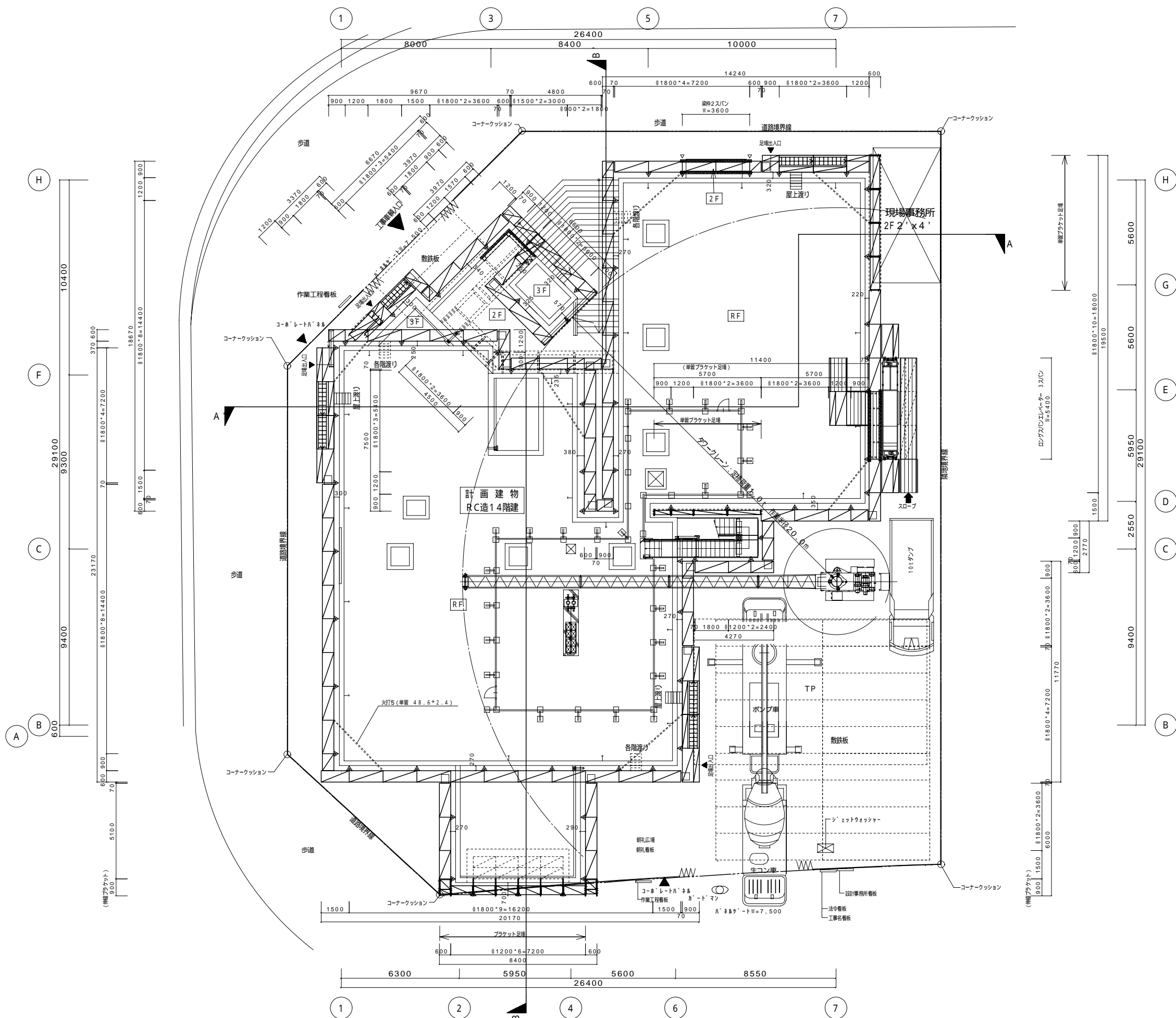
足場平面計画図 S = 1 / 100
